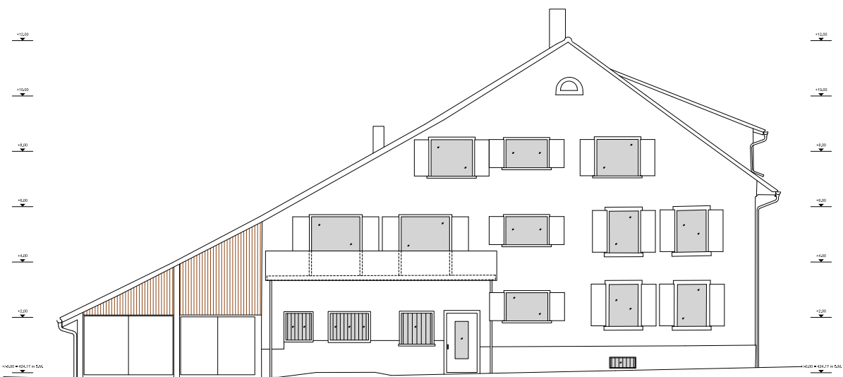
Ausschnitt Fassadenansicht 1:100
